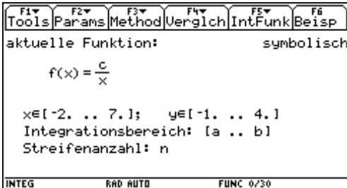
Das Integral von c x^{-1}
