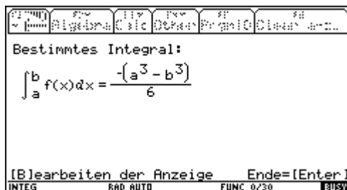
Bestimmtes Integral mit \circ \tilde{o}
