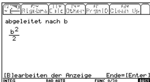
Ableitung nach b
