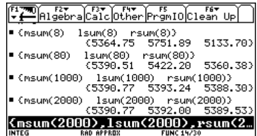
Für n = 2000 gibt's längere Rechenzeiten!
