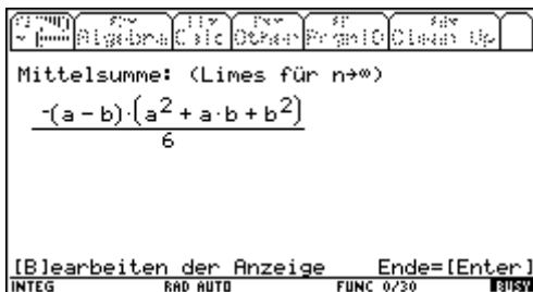
Berechnung des Limes mit \circ \tilde{m}
