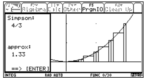
Simpson-Verfahren mit n = 4
