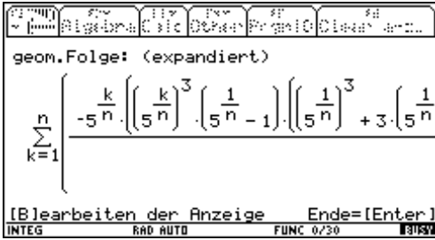
So sieht die Summe aus
