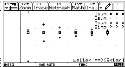
Grafik zur nebenstehenden Matrix
